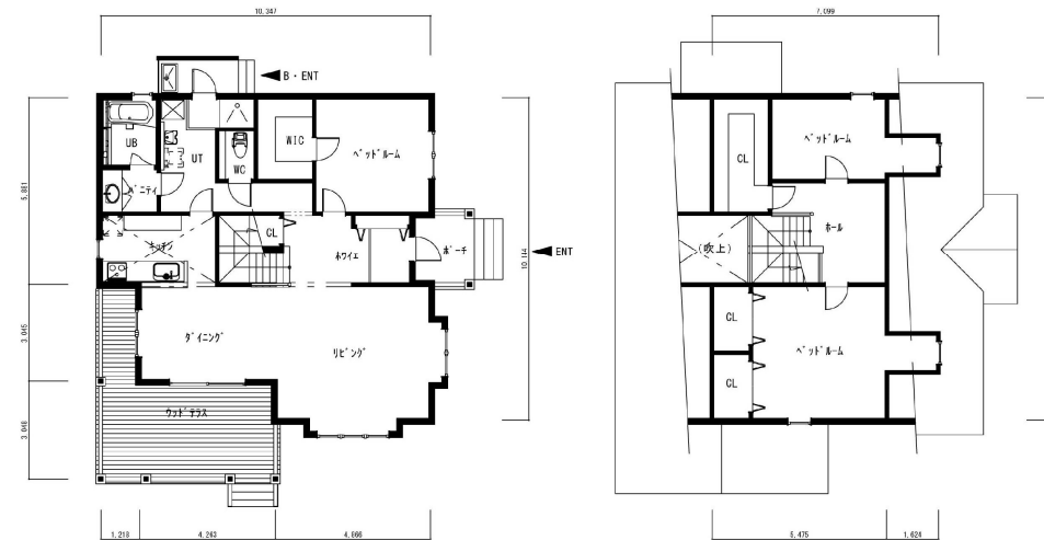
1 階平面
