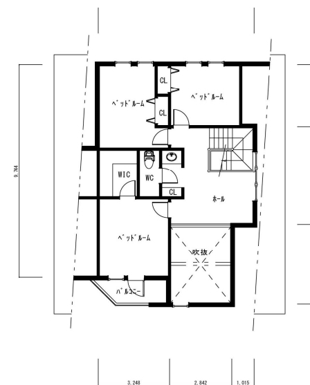
2 階平面
