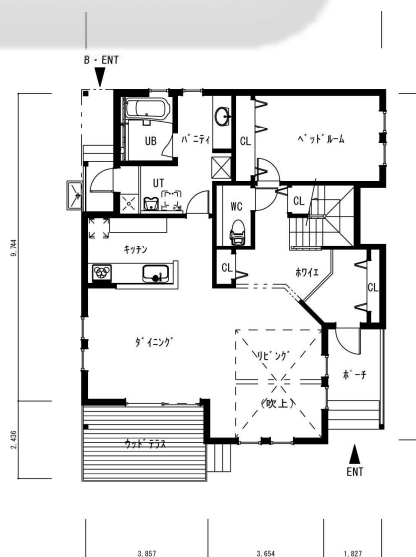
1 階平面
