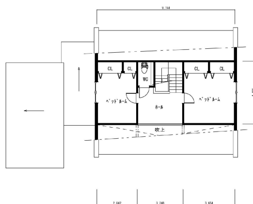
2 階平面
